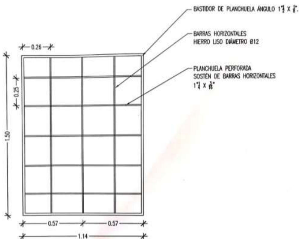
PROPUESTA REJA DE PROTECCIÓN 6º PISO HALL DE CASA DE GOBIERNO - 5 UNIDADES
